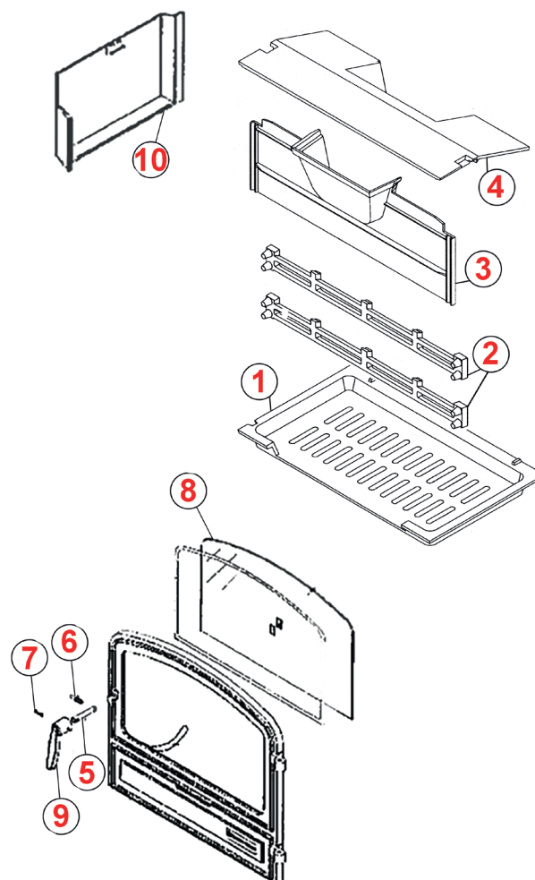
10 BRIQUE GAUCHE LINKERSTEEN 1341201050 FB 305015-00
