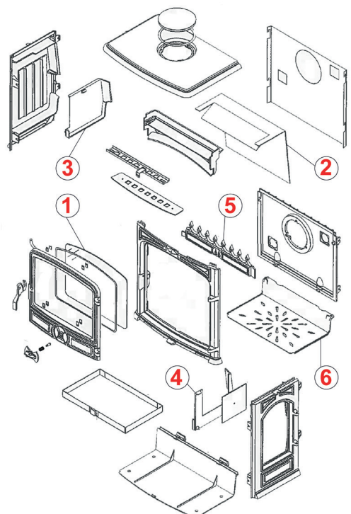
4 BRIQUE DROITE RECHTERSTEEN 1340803052 FB 305213-00
