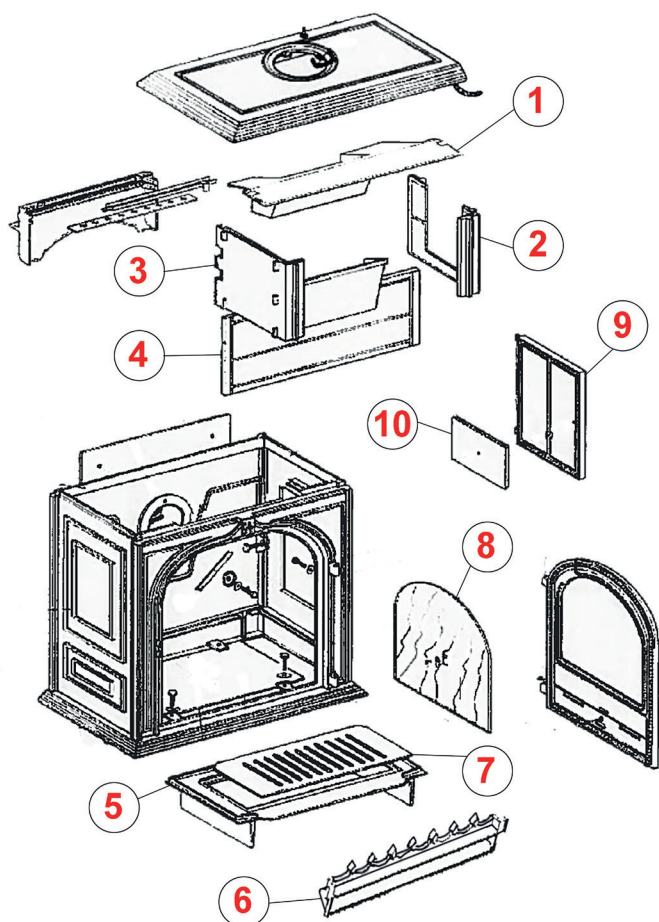
9 PORTE LATÉRALE ZIJDEUR 134100150 FB 303510-00
