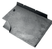
6 1390.52 FB 305202 BRIQUE ARRIÈRE DROITE ACHTERPLAAT RECHTS
