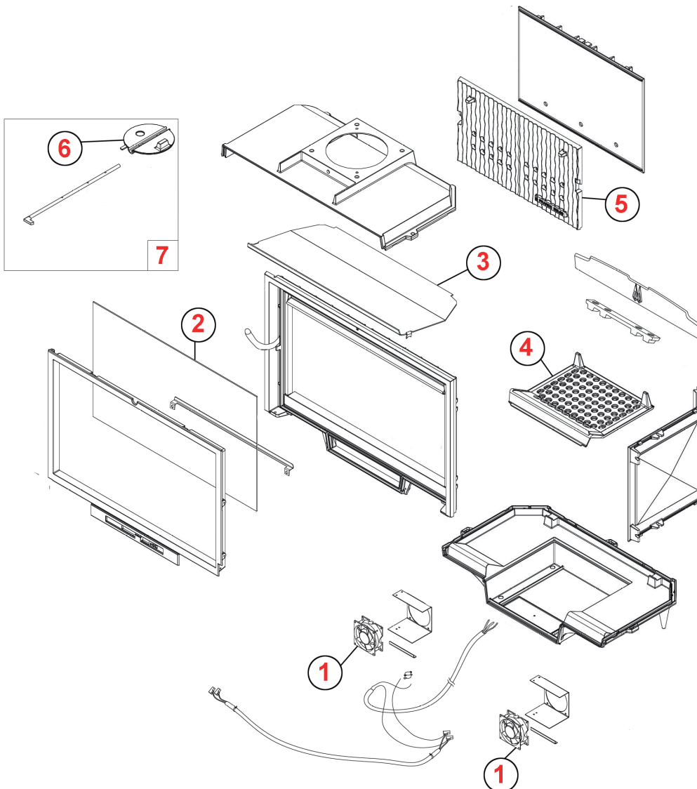
5 PLAQUE MOTIF ACHTERPLAAT 634134 FB330015-00
