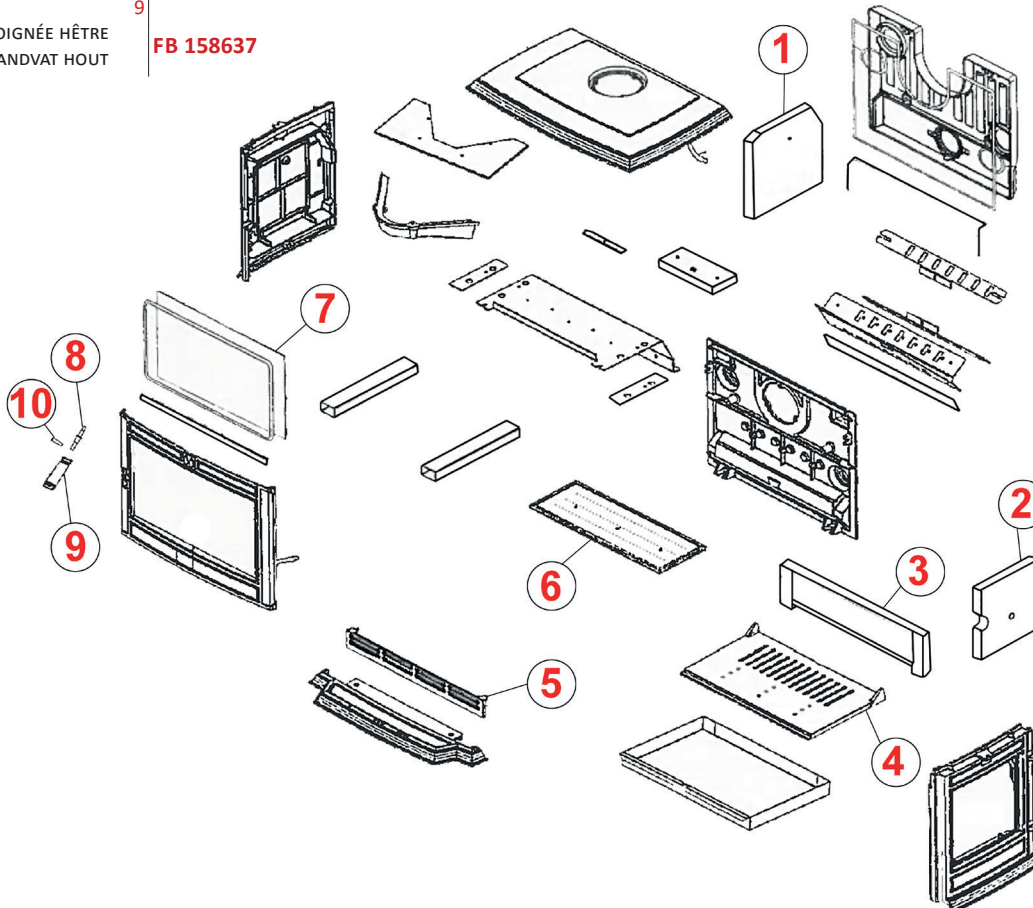
10 GOUPILE ÉLASTIQUE ELASTISCHE PIN 4mm*16mm FB 134758
